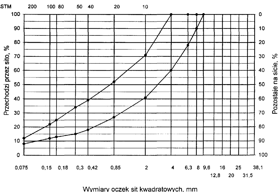
Rys. 1. Krzywe graniczne uziarnienia mieszanki mineralnej BA od 0 do 16mm, od 0 do 12,8 mm do warstwy ścieralnej nawierzchni drogi o obciążeniu ruchem KR1 lub KR2
